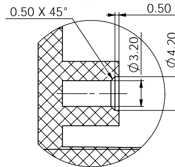
局部视图 E 比例 3:1
