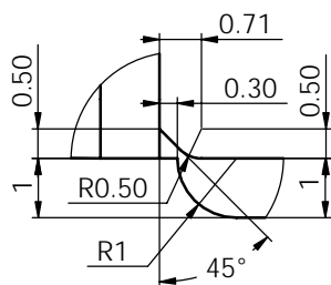
局部视图 B 比例 10:1
