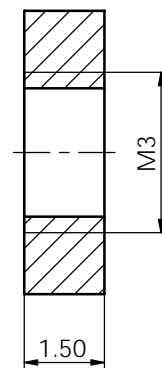
剖面 A-A
