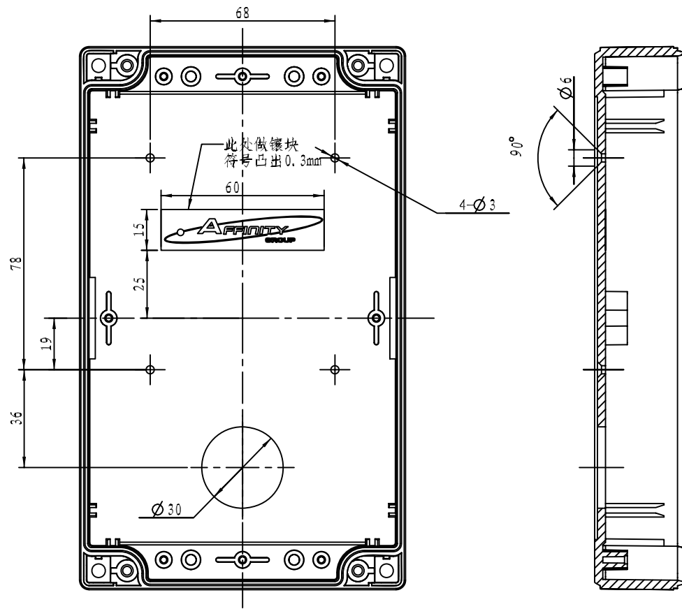
剖面 A-A
