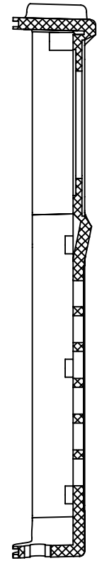
剖面 A-A
