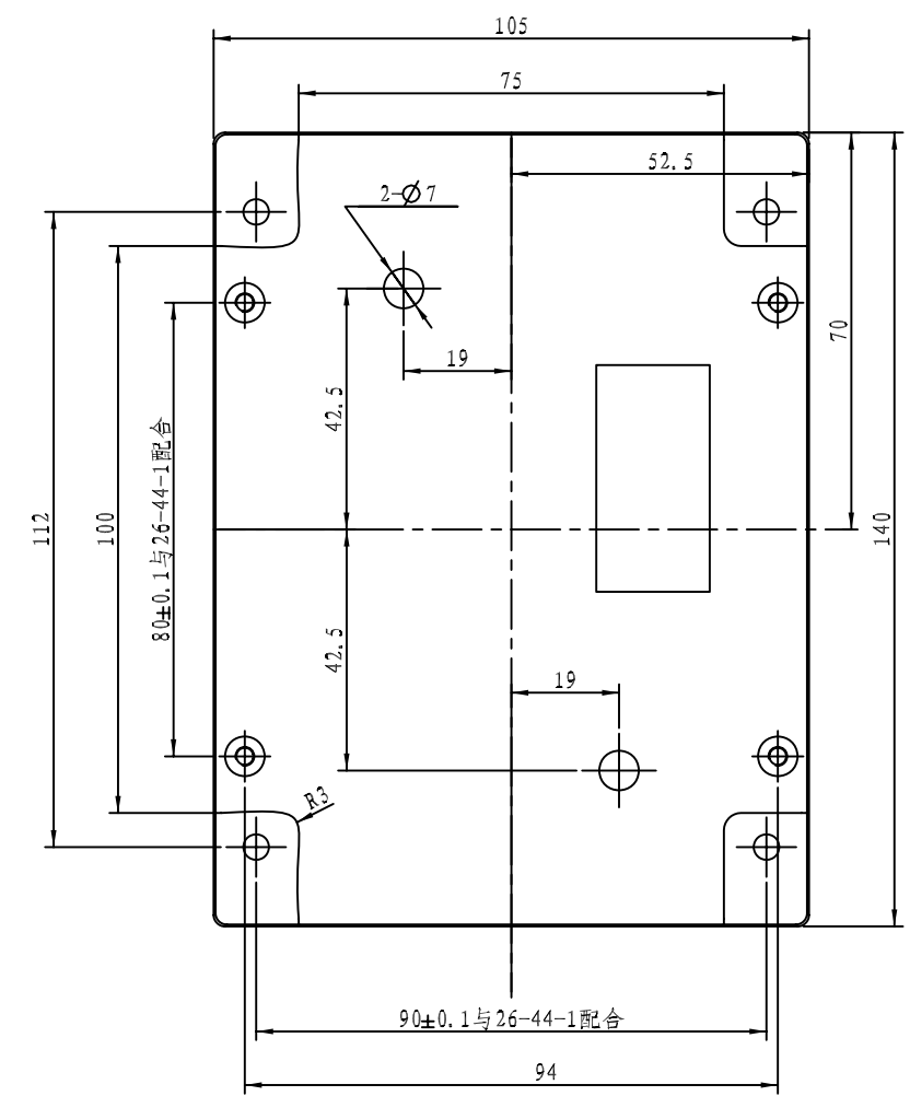
正面 (外表面)
