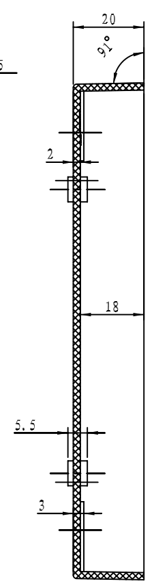
剖面 A-A
