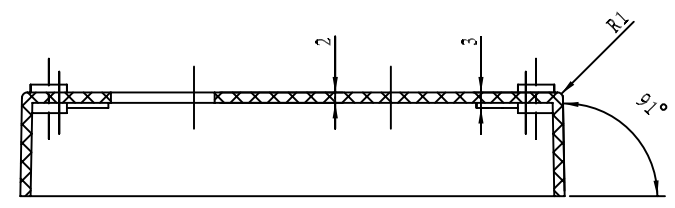
剖面 B-B
