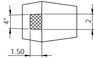
剖面 A-A
