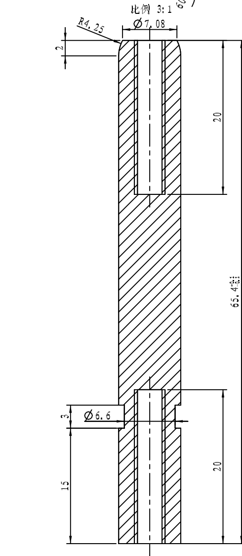
剖面 A-A
