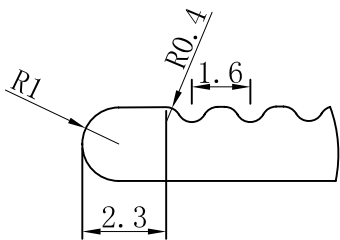
局部放大图A 5:1
