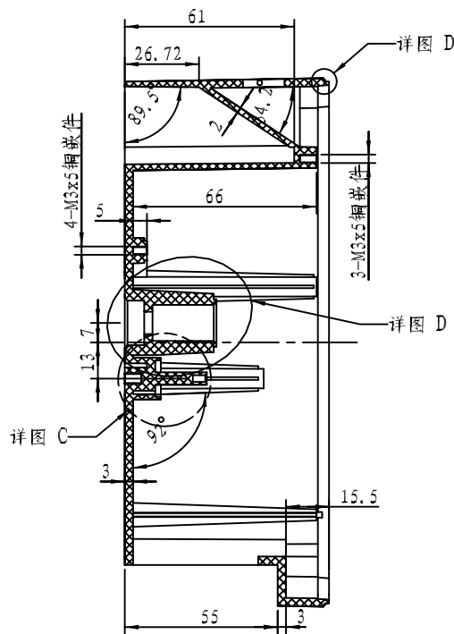
截面 A-A
