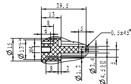
细节 C 刻度 1:1
