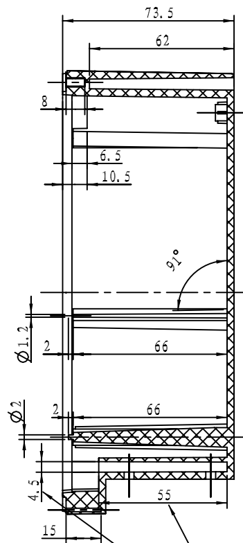
截面 B-B
