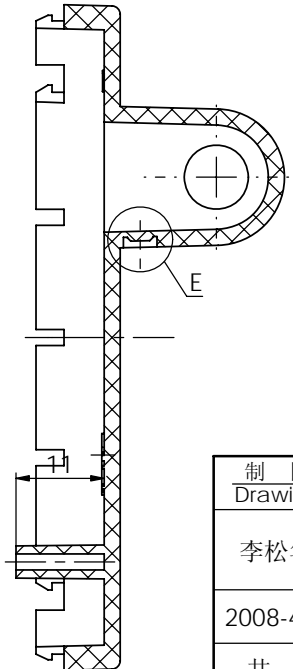
剖面 D-D
