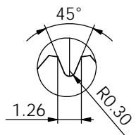
局部视图 B 比例 5:1
