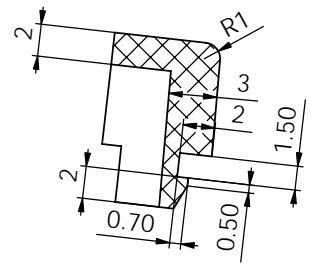
剖面 C-C 比例 3:1
