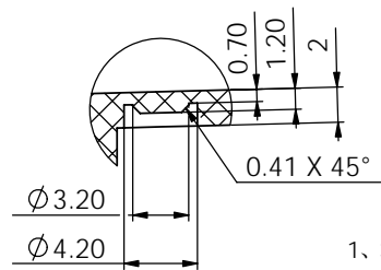
局部视图 E 比例 3:1
