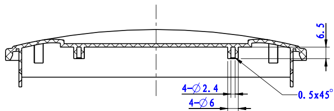
截面 A-A
