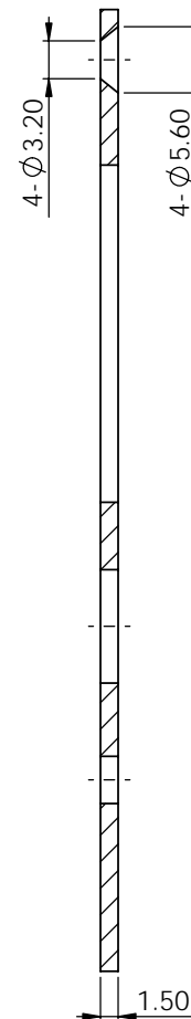
剖面 A-A
