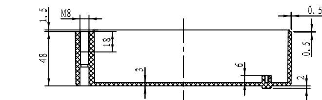
截面 A-A
