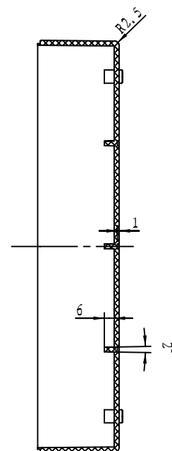
截面 B-B
