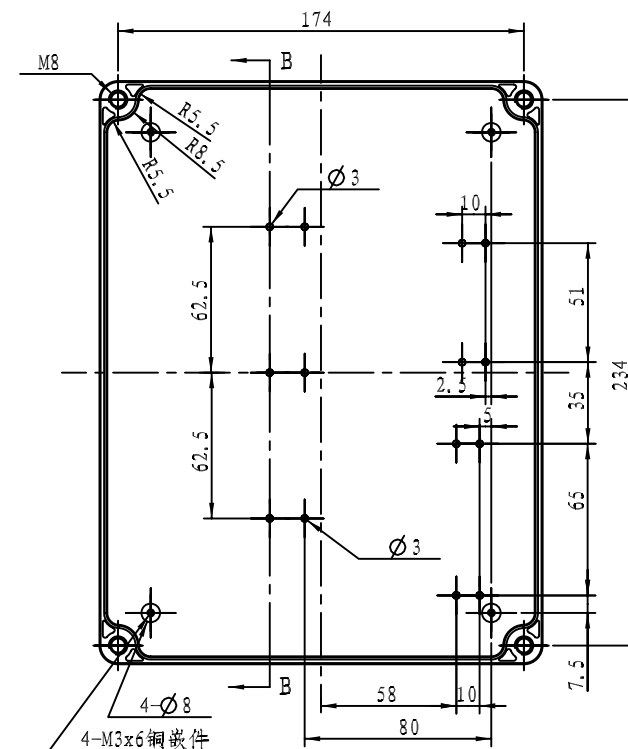
背面(顶杆做此面)
