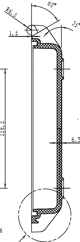
剖面 A-A
