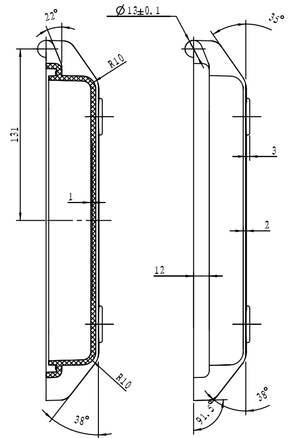
剖面 C-C
