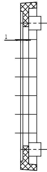
剖面 B-B
