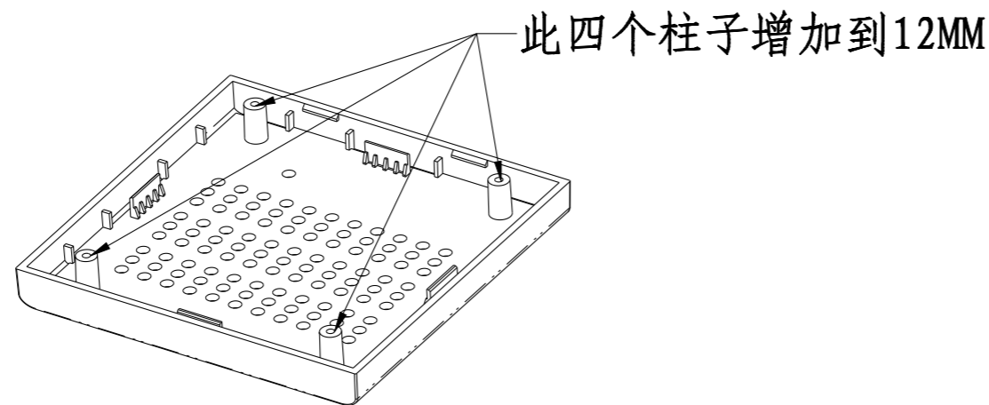
比例 1:2
