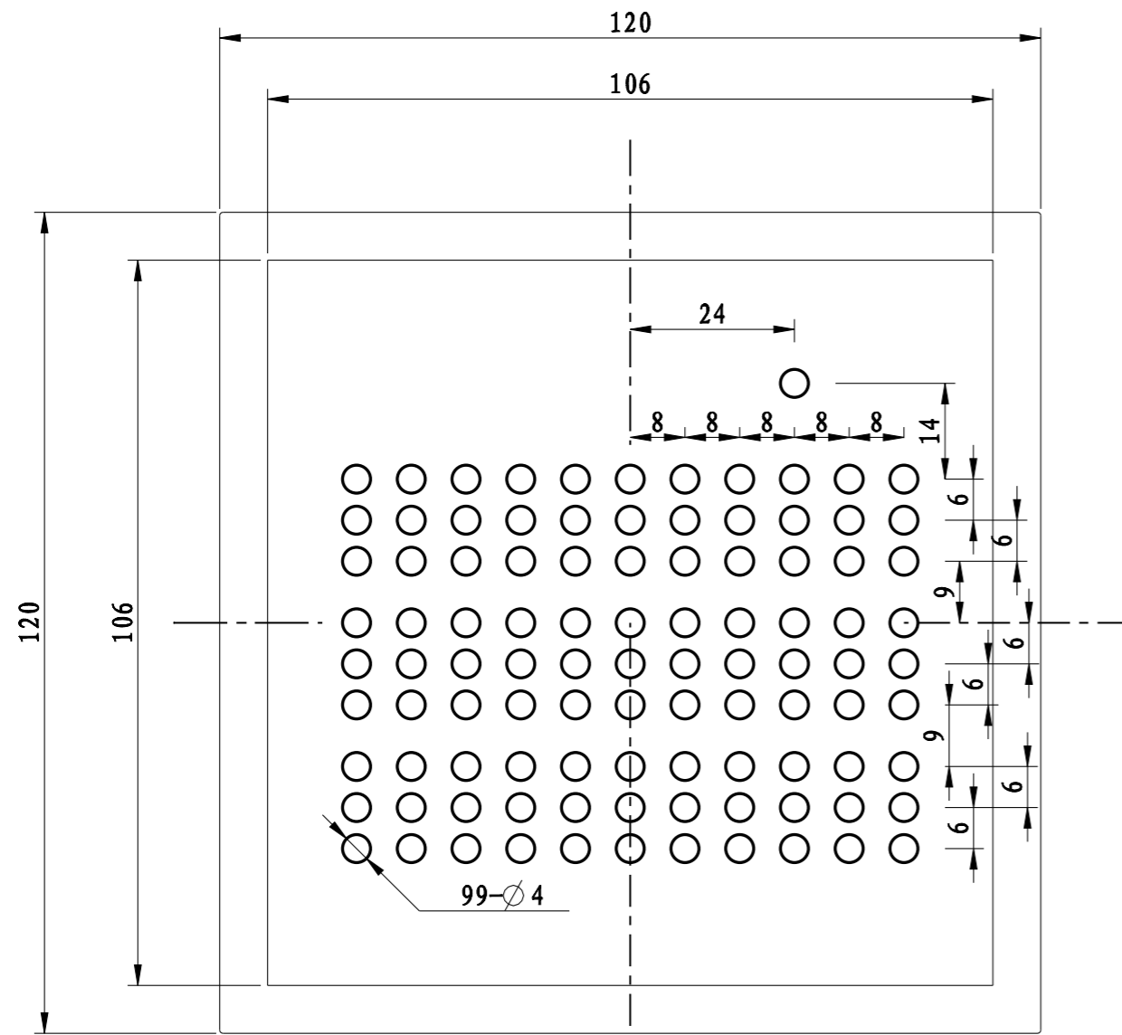
比例 1:1
