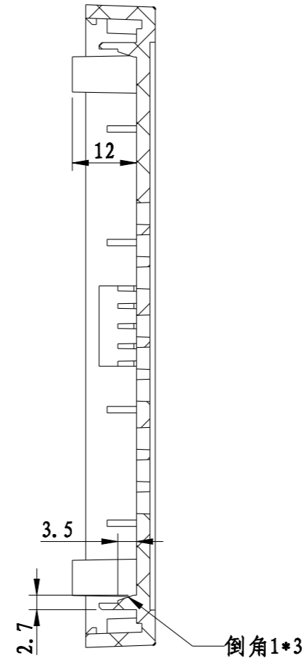
截面 A-A
