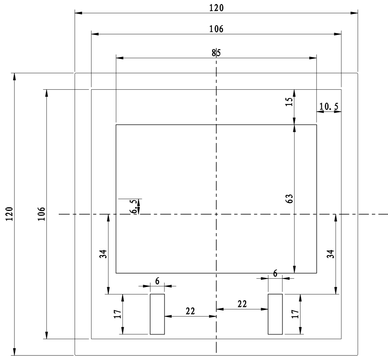
比例 1:1
