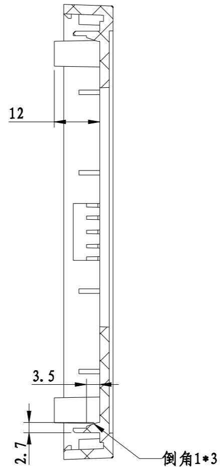
截面 A-A
