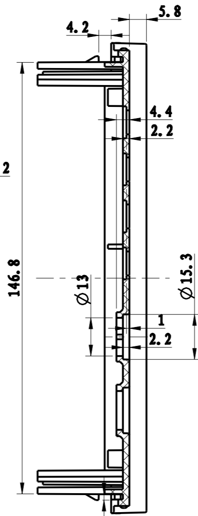
剖面 C-C
