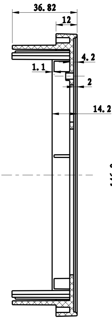
剖面 B-B
