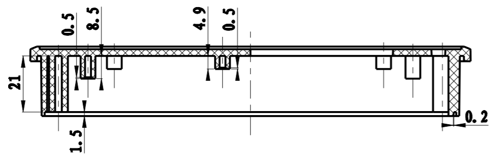
剖面 B-B
