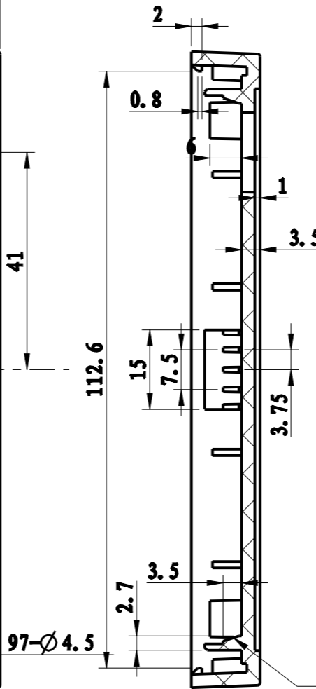
截面 A-A
