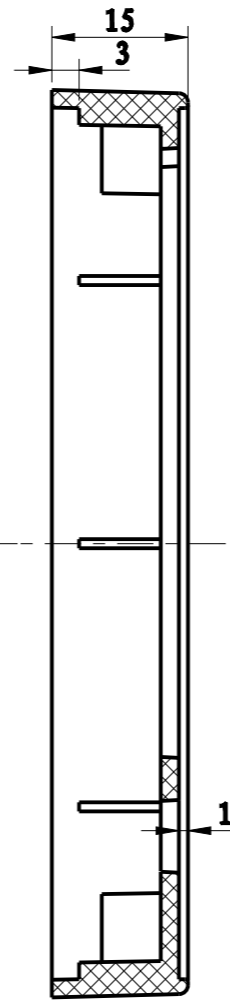
截面 A-A
