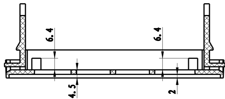
截面 A-A
