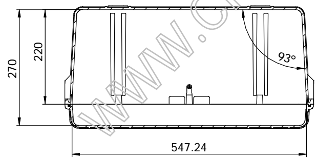
剖面 C-C
