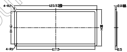
配15-11机箱平面板:
