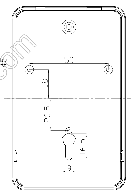
下盖正视图
