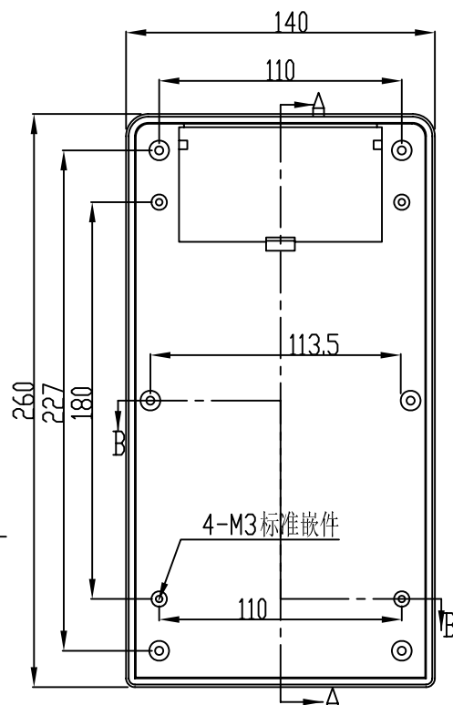
下盖反面视图
