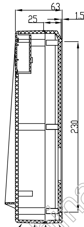
下盖 上盖
