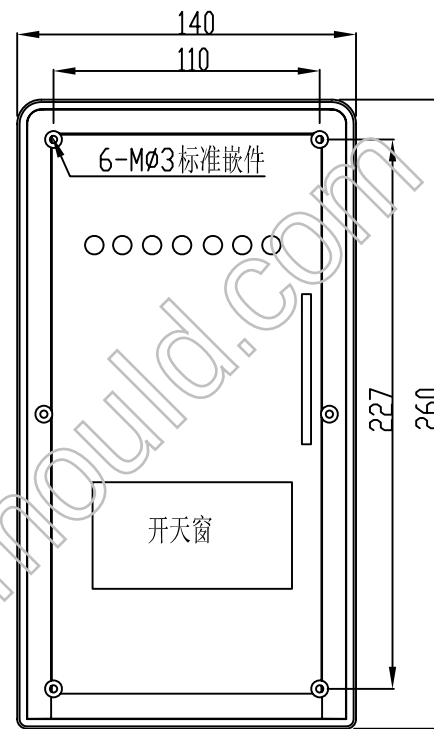
下盖反面视图
