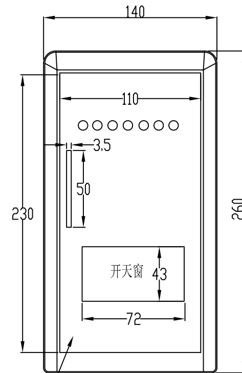
下盖正面视图
