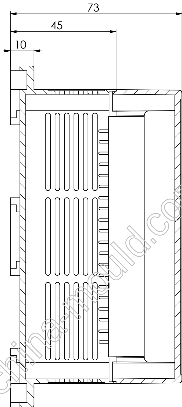
剖面 A-A
