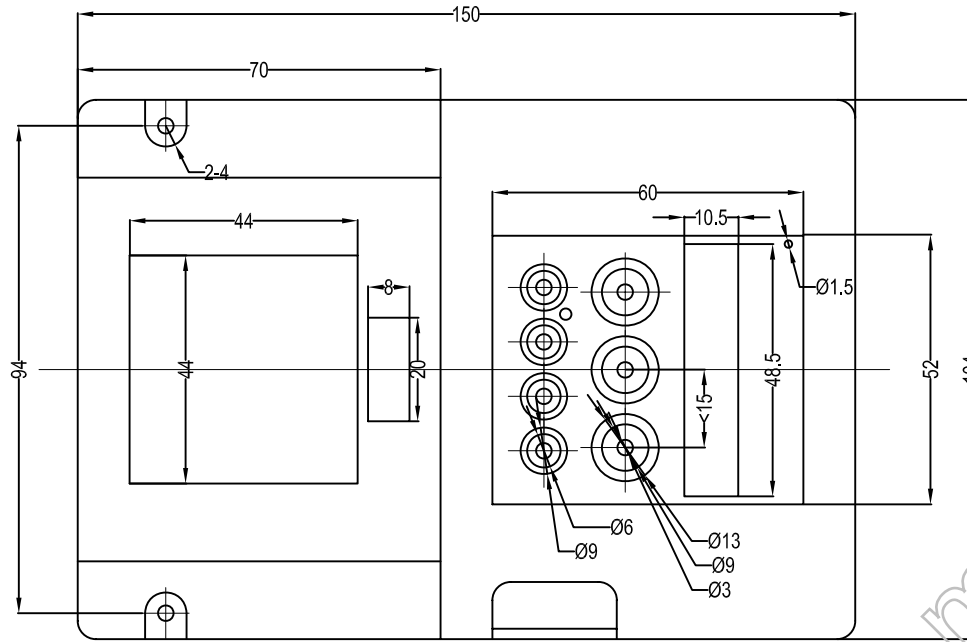
A向正面图
