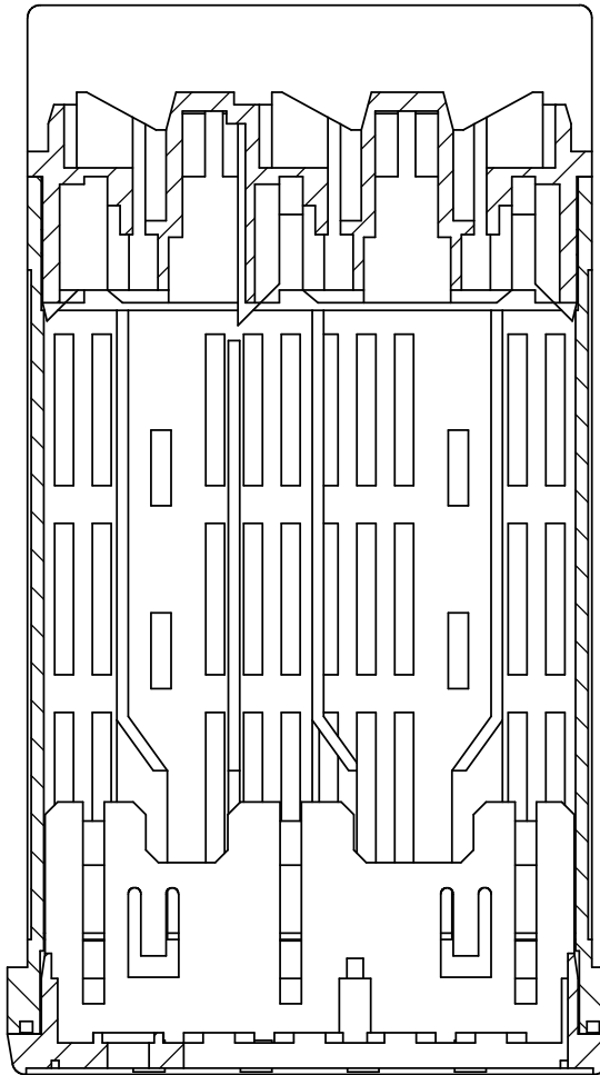
剖面 A-A
