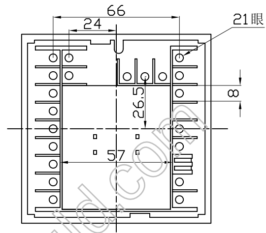
底视图
