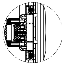
手柄安装剖面图
