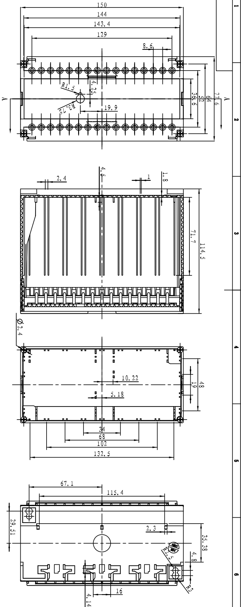
剖面 A-A
