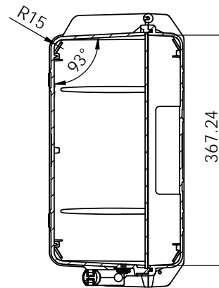
剖面 A-A
