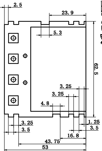
上PCB板
