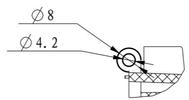
细节 A 比例 4:5
