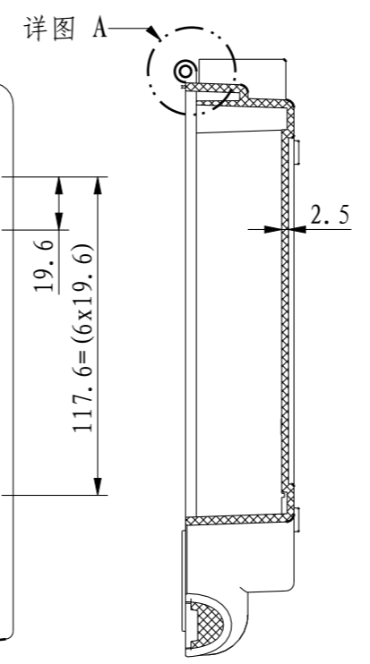
截面 A-A
