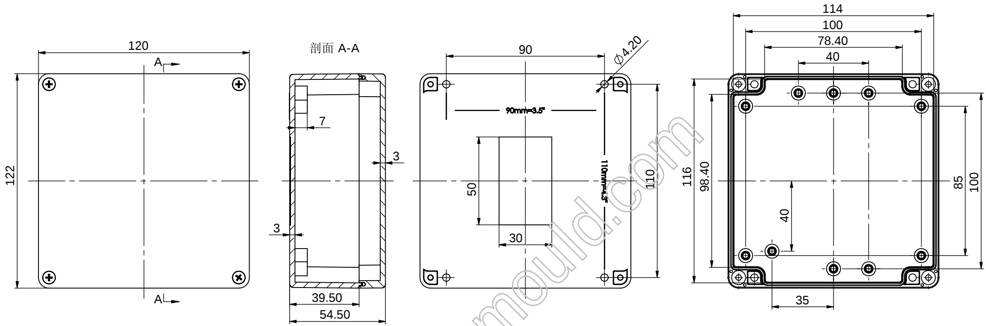
底壳内部图
